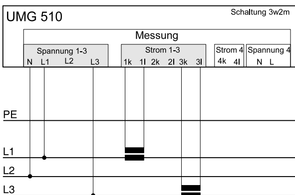
Abb.: 4.6 Dreiphasige Messung ohne Nullleiter in Aronschialtung (3w2m).
