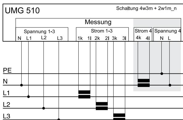
Abb. 4.13: Messung im Vierleiternetz mit Hauptmessung (Abb.4.1) und Hilfsmessung (Abb.5.4).
