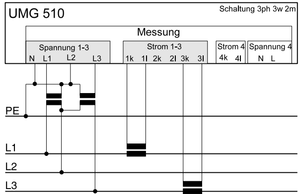
Abb. 4.6a Dreiphasige Messung ohne Nullleiter in Aronschialtung mit Spannungswandlern (3ph 3w 2m).
