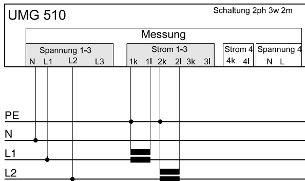
Abb. 4.9: Zweiphasige Messung für Netze mit 180° Phasenverschiebung zwischen L1 und L2 ( 2ph 3w 2m ).
