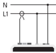
Einphasig
