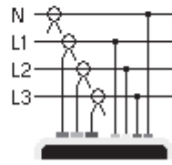
Dreiphasig 4 Leiter
