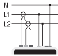
Zweiphasig
