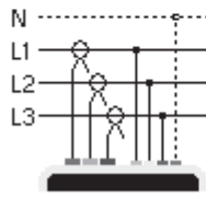
Dreiphasig 3 Leiter
